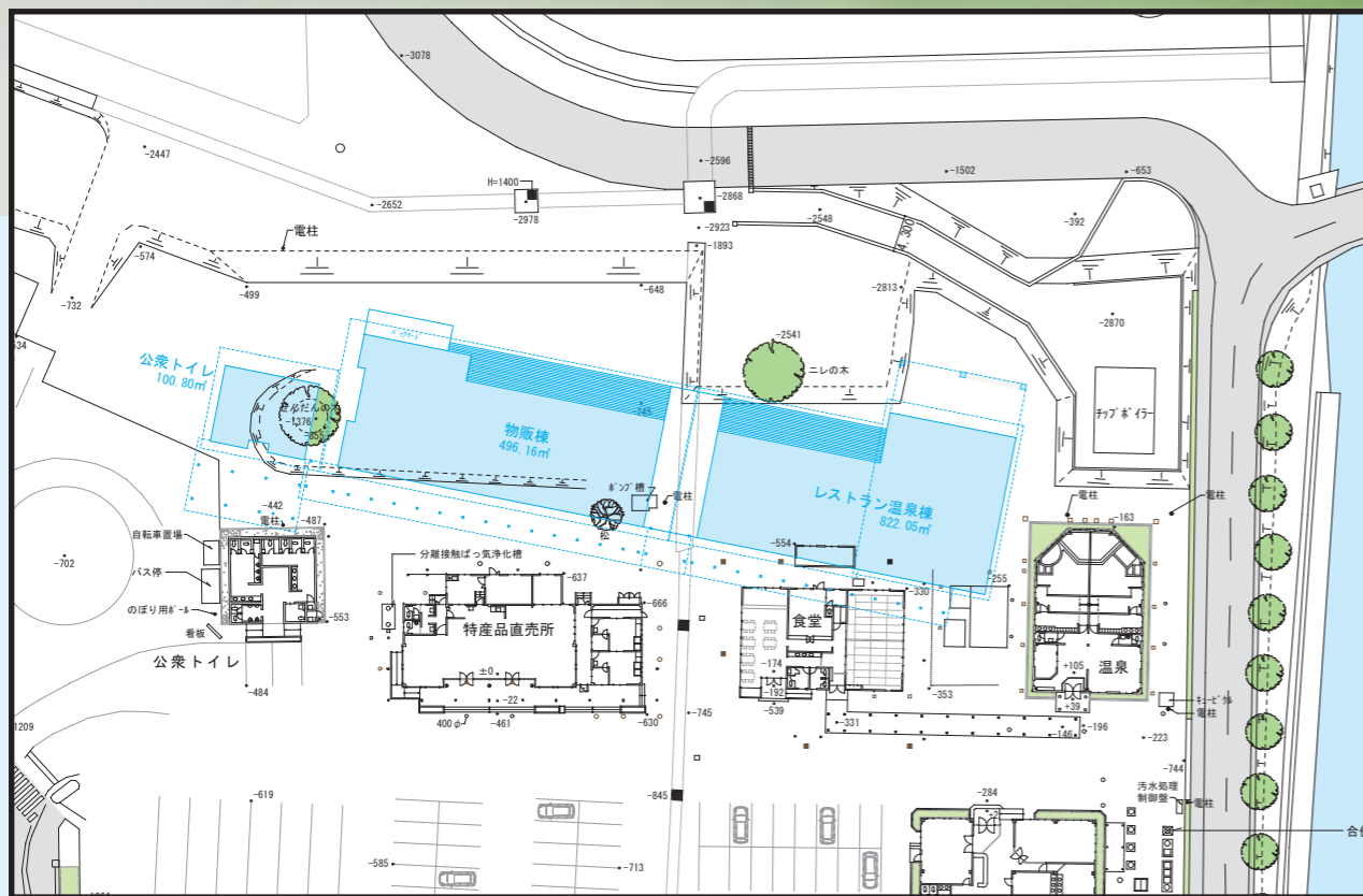
(配置図) 現在地との比較.....青色の建物が新しい道の駅
